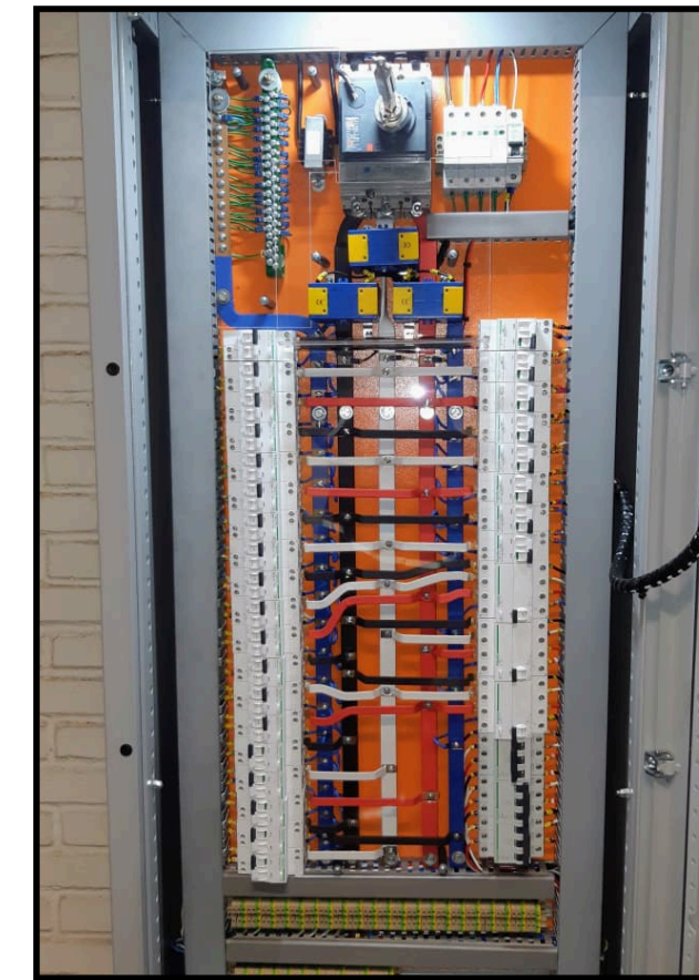
Montagem de quadros elétricos
